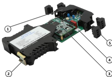
图 1.3 网关设备整机结构
